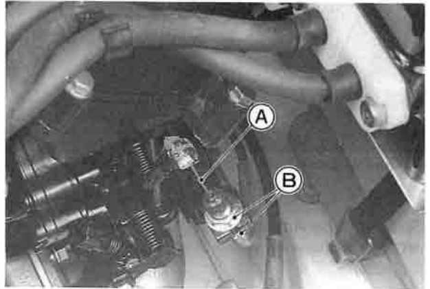
A. Choke Cable B. Locknuts
