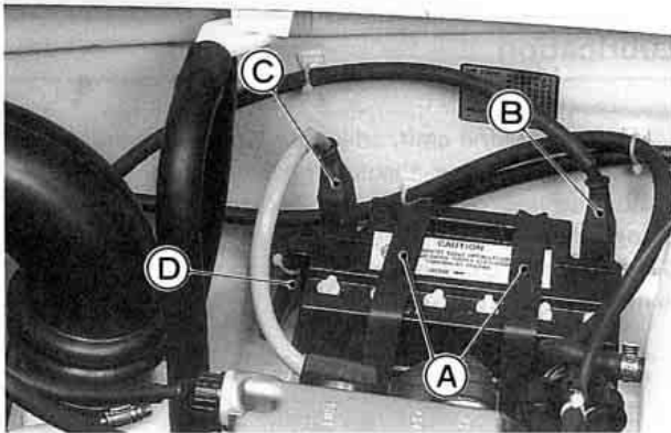
A. Straps
