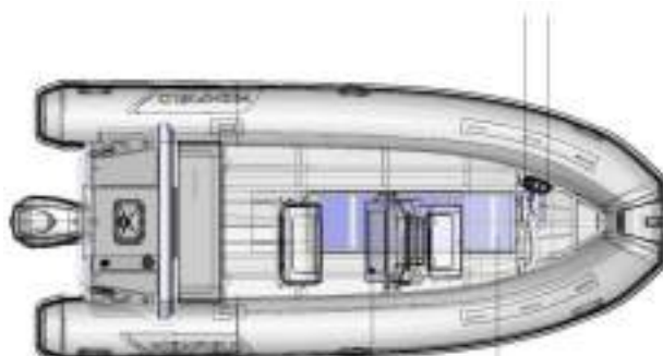
Darstellung Kraftstoffsystem
