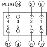
PLUG DETAIL H DEUTSCH DT06-8S
